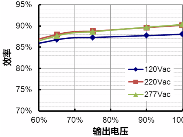
LUD-060S150BS2 (Io=1050mA) 效率 vs. 输出电压
