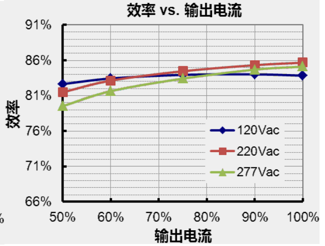
EUV-042S048PS 效率 vs. 输出电流
